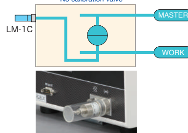
漏れ基準方式 Leak reference method
