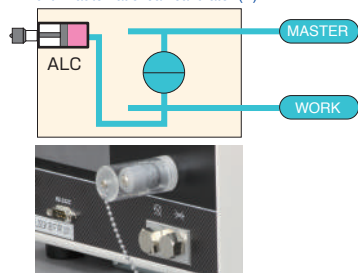
容積変化方式 Volumetric change method
