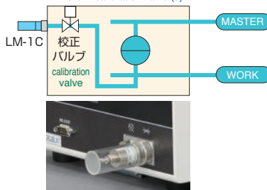
漏れ基準方式 Leak reference method
